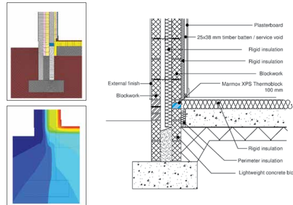
BRE detail 600023
