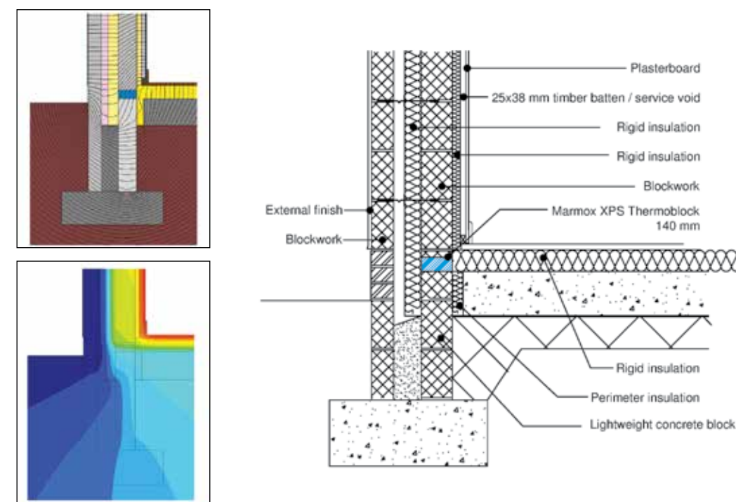
BRE detail 600024
